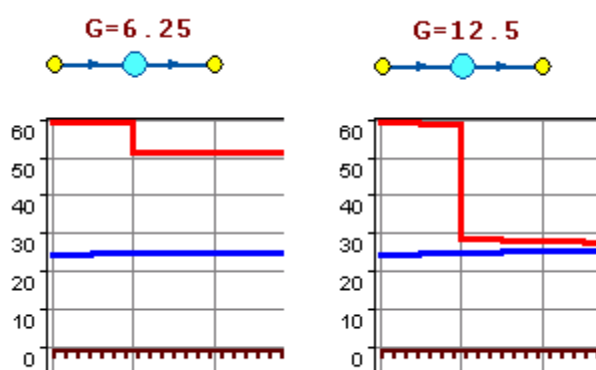
Рисунок 21 – Характеристики дроссельных шайб
