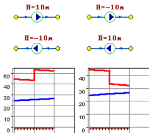
Рисунок 17 – Пьезометрические графики
