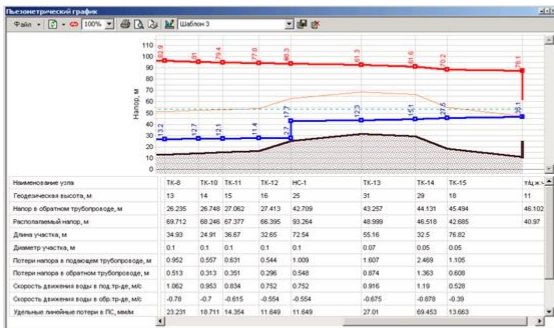
Рисунок 25 – Пьезометрический график
