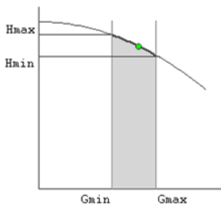
Рисунок 18 – Напорно-расходная характеристика насоса
