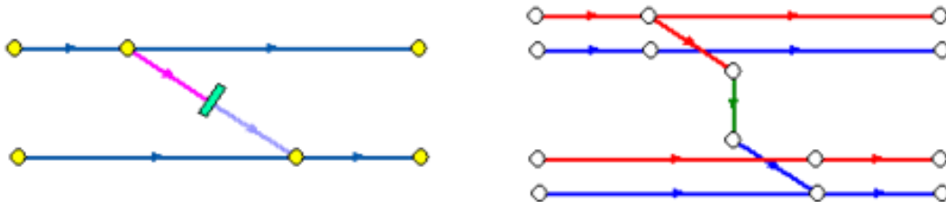
Рисунок 15 – Соединение между подающим трубопроводом одного участка и обратным трубопроводом другого участка
