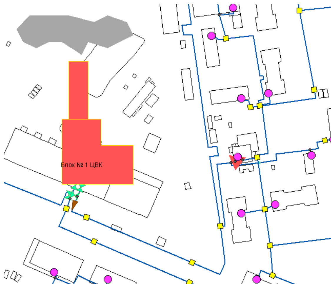
Рисунок 28 – Фрагмент схемы тепловых сетей
