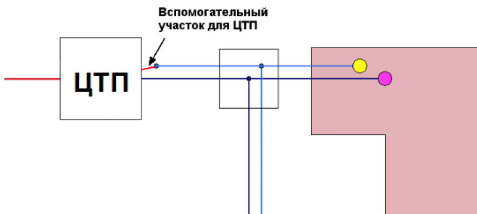
Рисунок 7 – Подключение трубопровода ГВС
