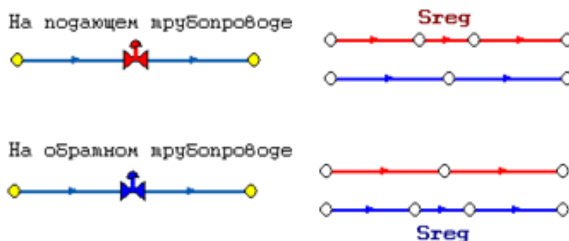
Рисунок 19 – Дросселирующие устройства
